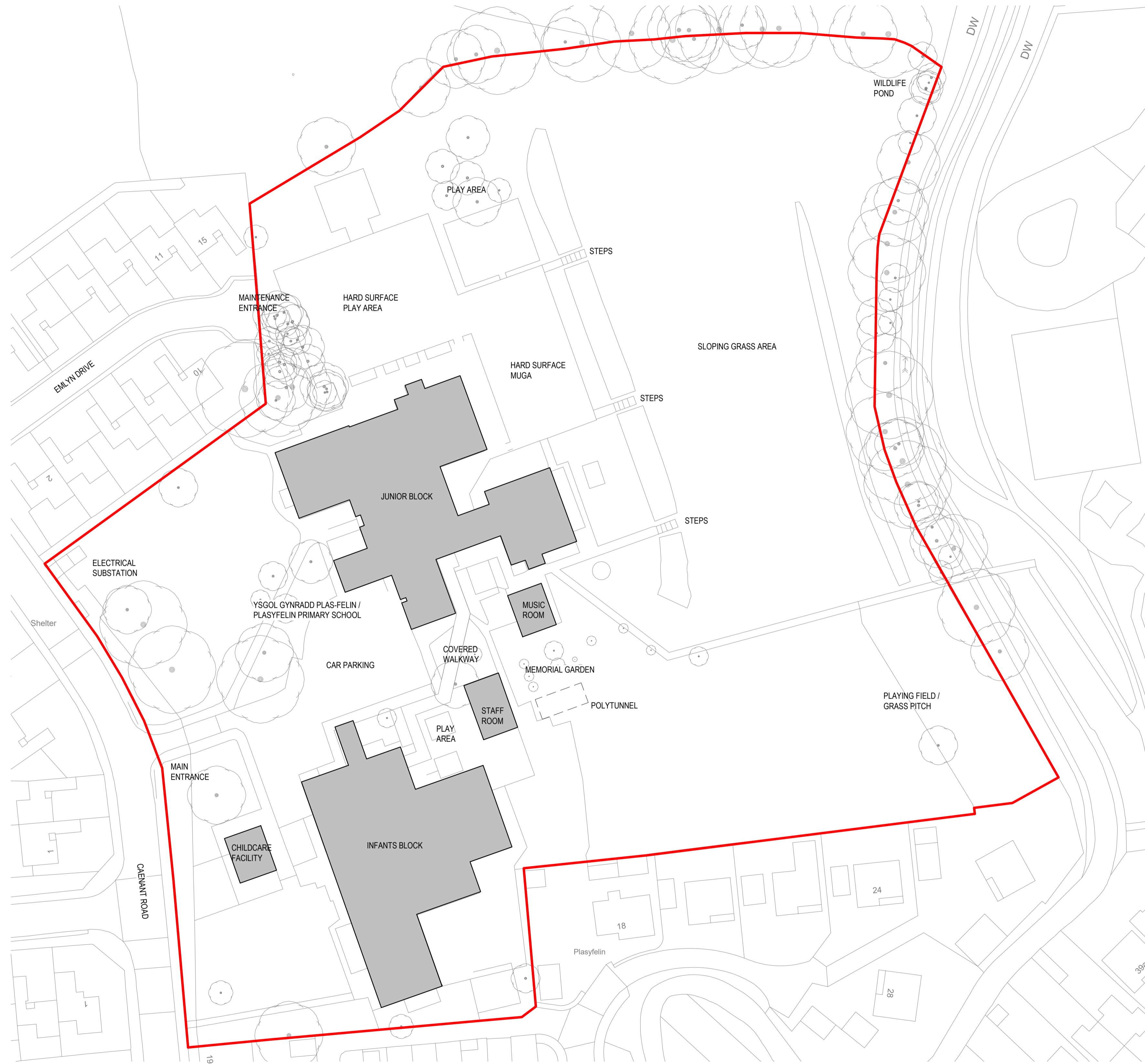
EXISTING SITE PLAN 1 : 500
