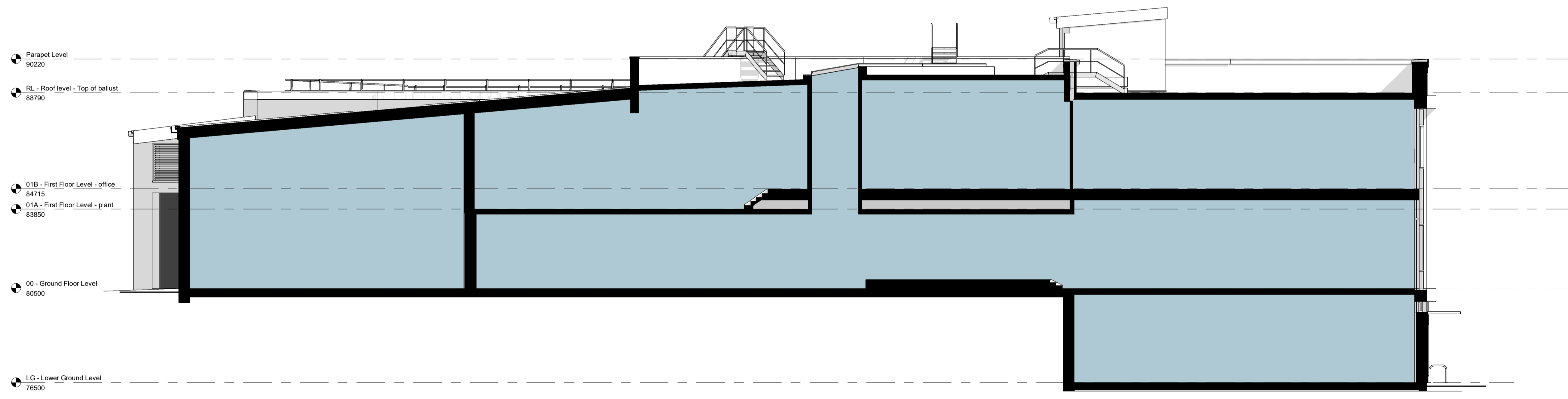
B Section B 1 : 100
