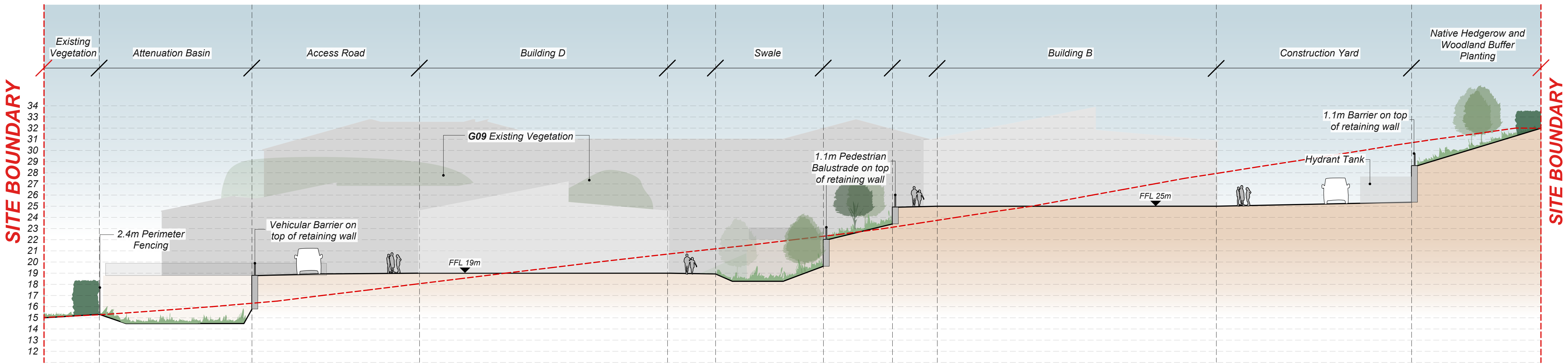
1 Section: A-A' Scale: 1:200
