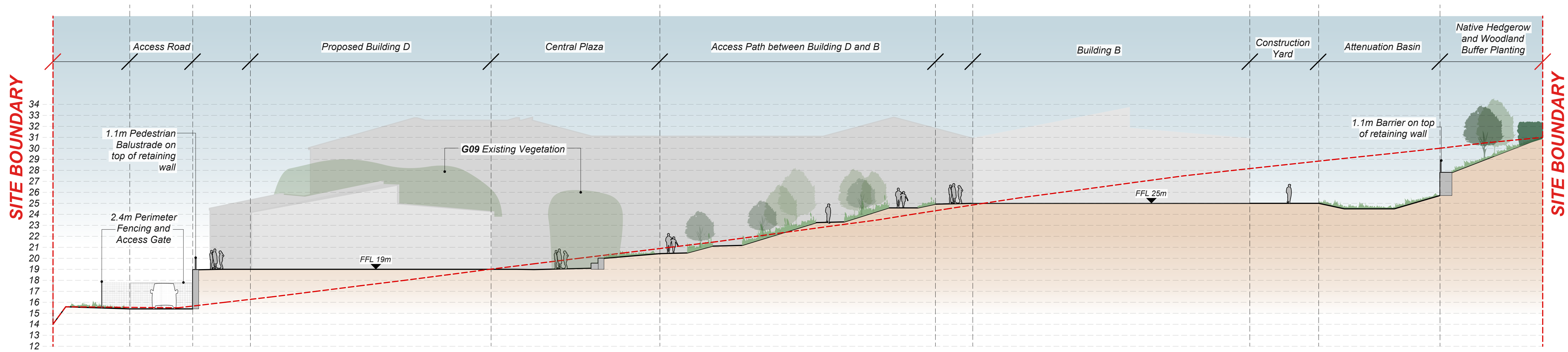
2 Section: B-B' Scale: 1:200
